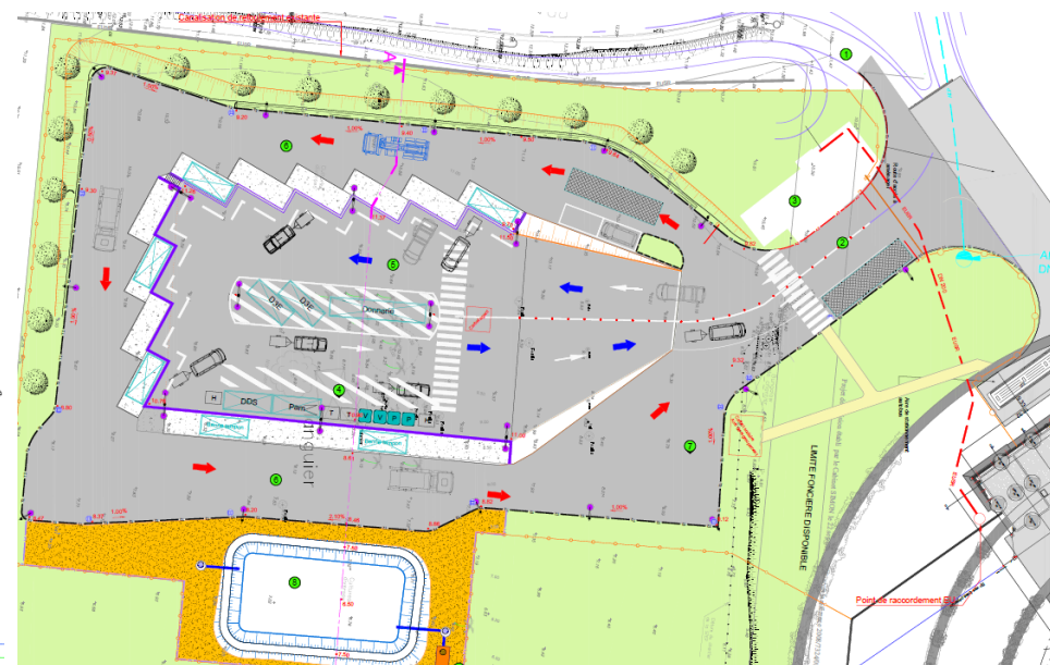
Vue en plan de l'aménagement
